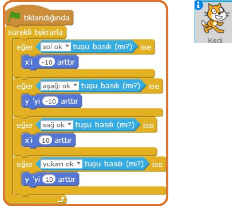
Şekil 101: Kedi kuklası yön tuşları ile hareket ettirme komutları
