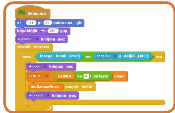
Şekil 117: 4 nolu tuşun komutları
